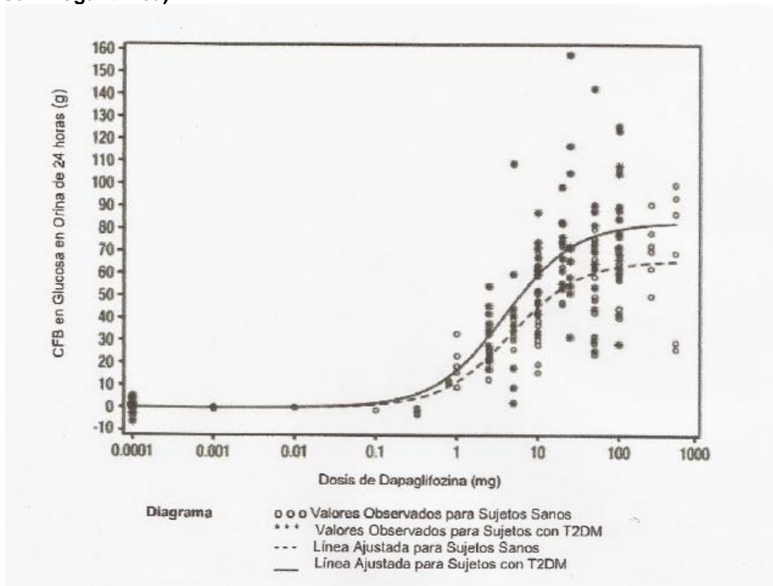
Figura 1: Diagrama de dispersión y Línea Ajustada de Cambio desde el Estado Basal en Cantidad de Glucosa en Orina de 24 horas versus Dosis de Dapagliflozina en Sujetos Sanos y Sujetos con Diabetes Mellitus Tipo 2 (T2DM) (Representación semi-logarítmica)
