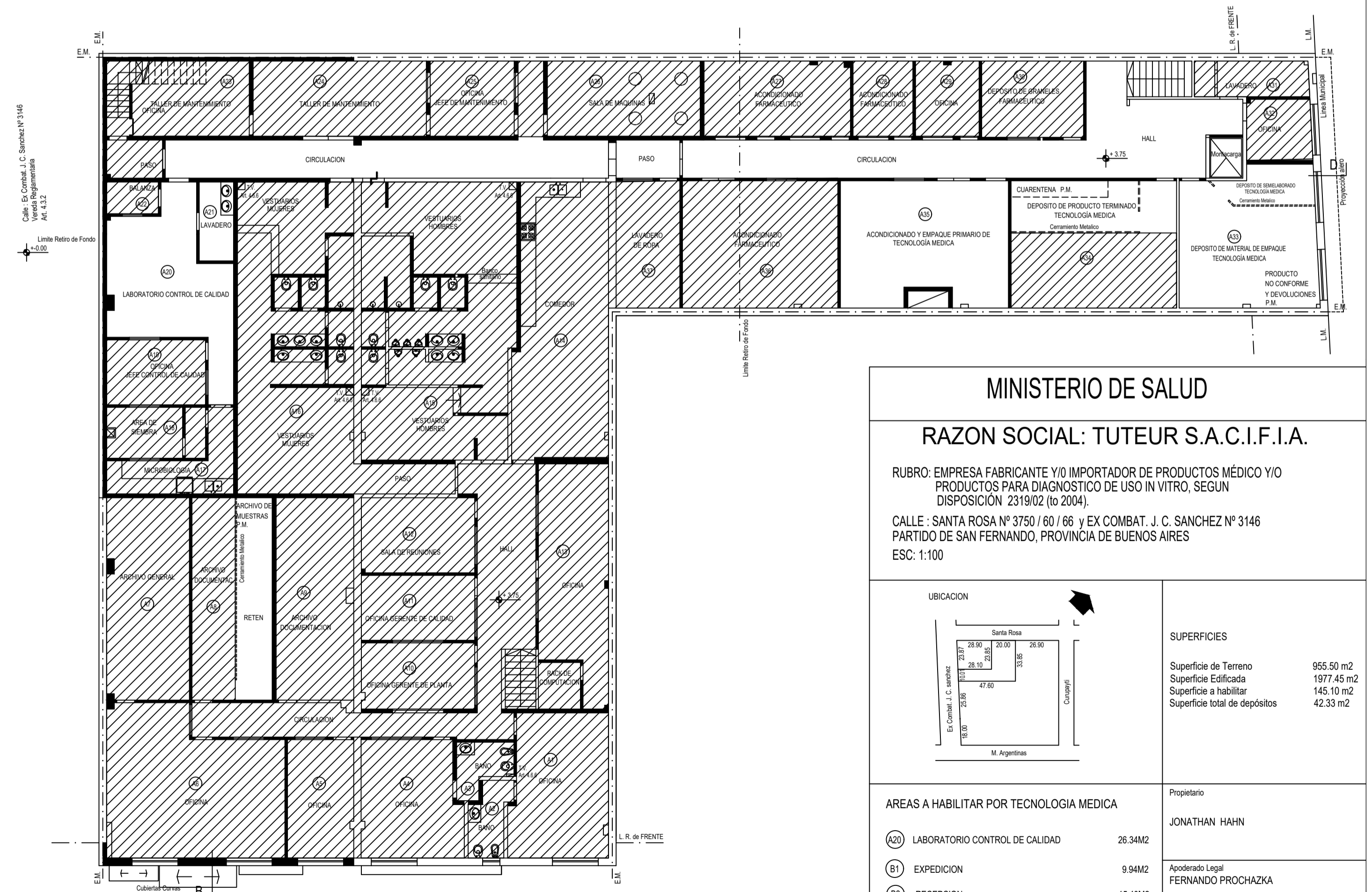
PLANTA 1º PISO
