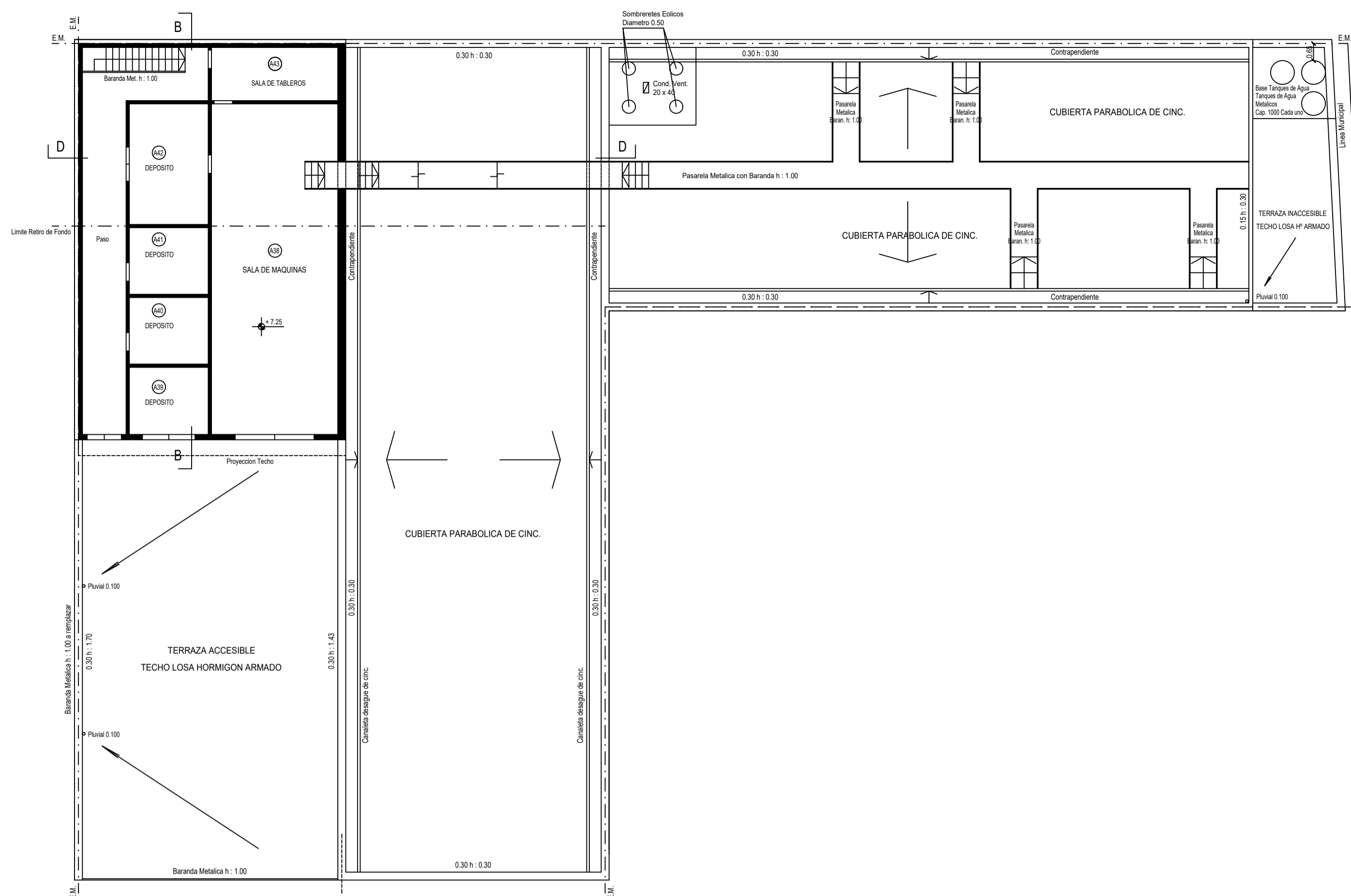
PLANTA 2º PISO y PLANTA DE TECHOS S / 1º PISO
