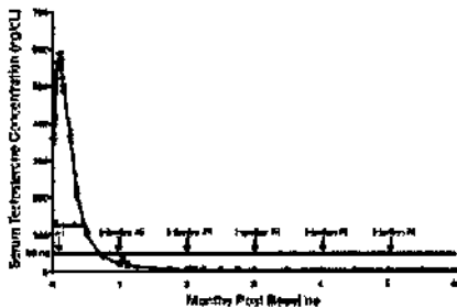
Figura 4. ELIGARD® 7,5 mg - Media de concentraciones séricas de testosterona (n = 117)
